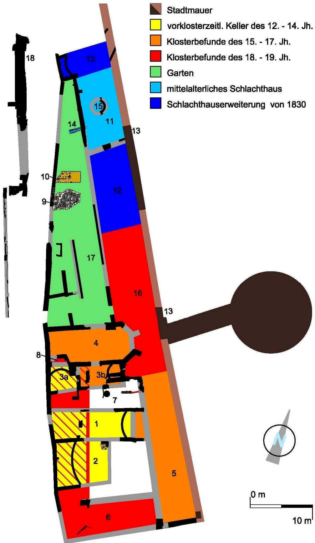
Plan 4, Übersichtsplan der Grabungsergebnisse östlich der Brückstraße mit dem bestehenden Kehlturm (schwarz) mit Ergänzungen (grau) und Rekonstruktion der Gebäude des Alexianerklosters und sonstiger Bauten (farbig)
